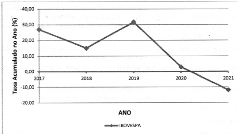
Gráfico 10 – Rentabilidade IBOVESPA (%) – 2017/2021
